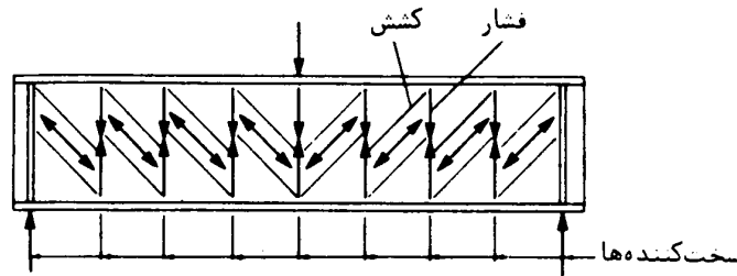
شکل ۳-۱۲ عمل میدان کششی
