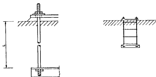
شکل ۱۲-۲۱ پیچ مهاري با نيشي مهاري [۱۴]
