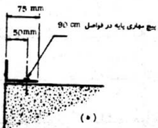
شکل ۸-۱۹ جزئیات انواع مختلف تکیه‌گاه پانل‌ها [۱۷]
