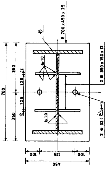
شکل ۱۲-۲۸ کف ستون نوع اقتباس از کارخانه ماشین سازی تبریز [۱۴]
