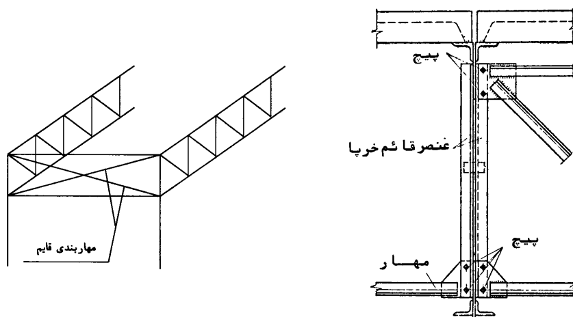
شکل ۹-۸-ب اتصال مهارهای قائم [۲]
