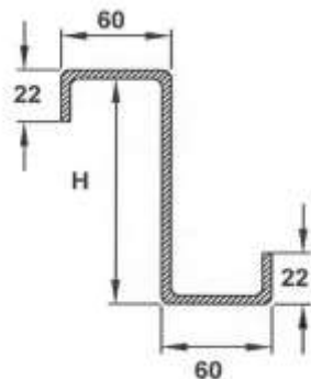
شکل شماره ۱ : پروفیل Z
